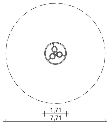
Zał. 1 Wymiary urządzenia i strefy bezpieczeństwa
