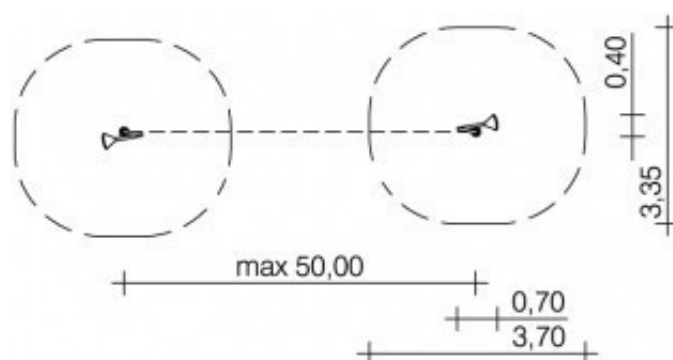
Zał. 1. Wymiary urządzenia i strefy bezpieczeństwa
